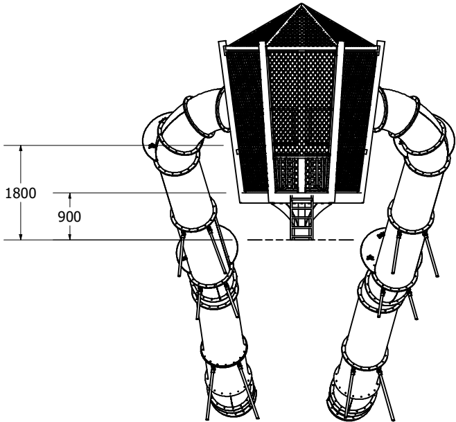
Right Elevation
