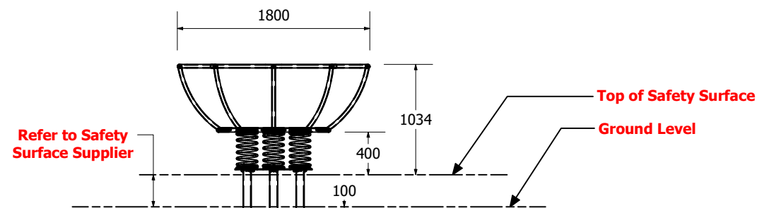
Right Elevation
