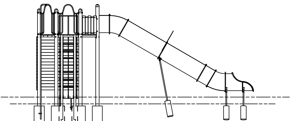
Right Elevation
