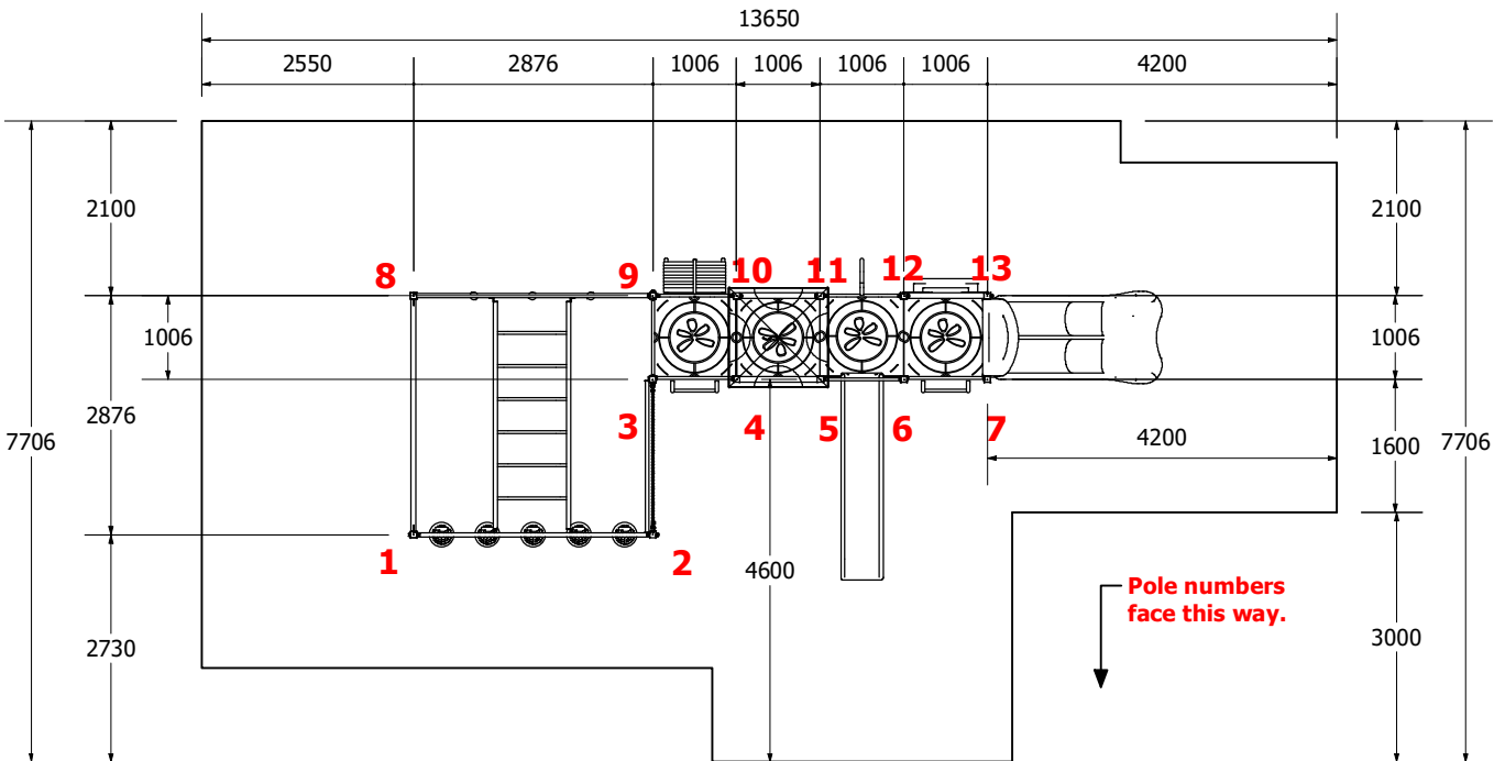
Pole Dimensions
