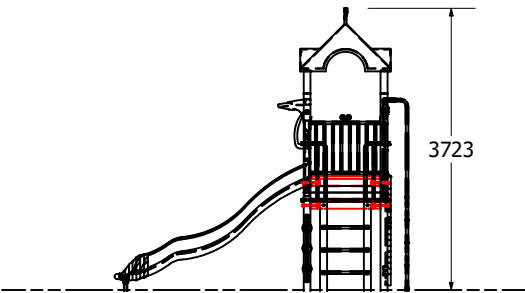
Right Elevation
