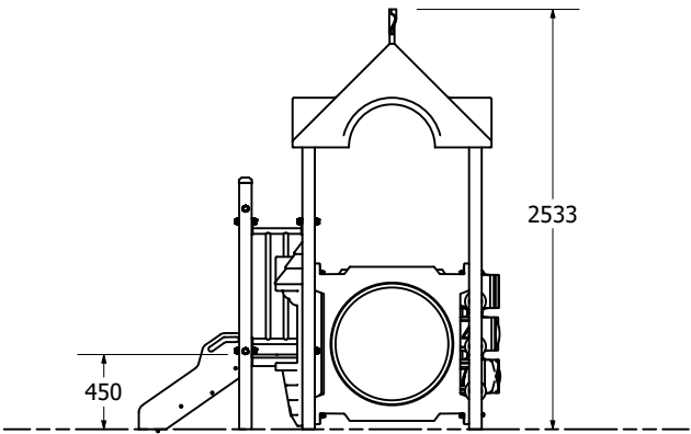
Right Elevation
